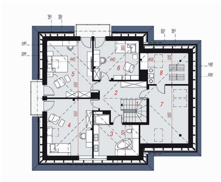
PODDASZE
