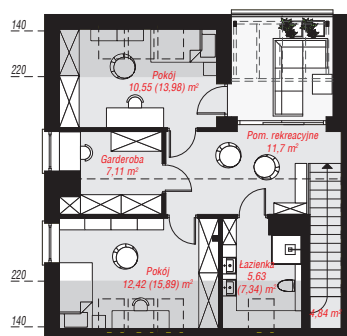
PODDASZE: 52,25 (60,86) m 2
