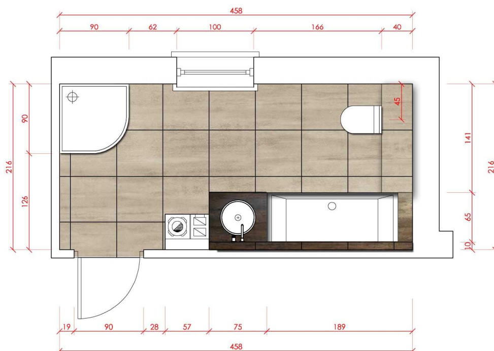
rzut/1:50
