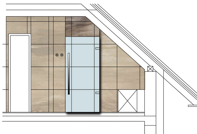
widok D/1:50
