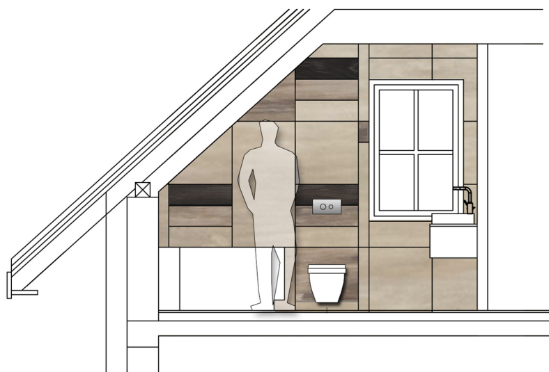
widok B/1:50
