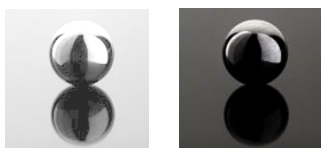
BIAŁY POŁYSK
