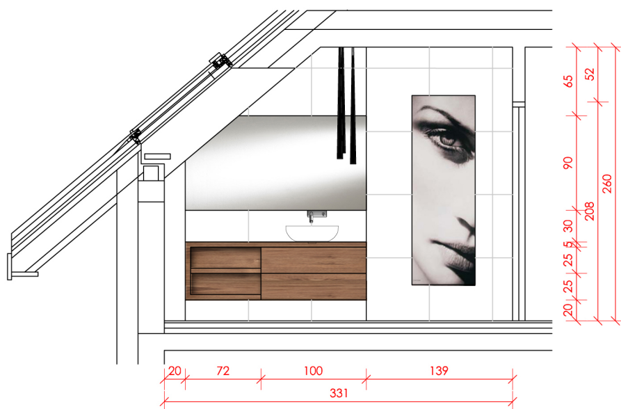
widok C/1:50
